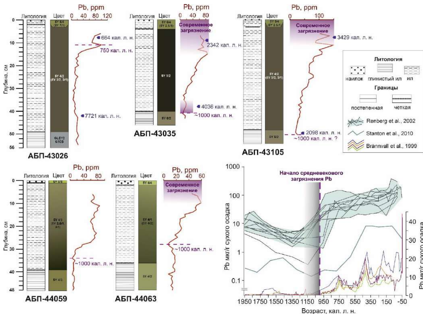
Рисунок 6 — Литологический состав изученных колонок и распределение концентраций Pb. Цвета обозначены кодами в соответствии с таблицей Munsell Soil Color Chart. Радиоуглеродные датировки обозначены синим цветом, Pb (изохроны) — лиловым. Затененные фиолетовые области на кривых Pb указывают на современное загрязнение Pb и неопределенности в начале средневекового загрязнения Pb. В нижней правой части представлено распределение Pb за последние 2000 лет на основе объединенных данных (Renberg et al., 2002; Stanton et al., 2010; Brännvall et al., 1999).
