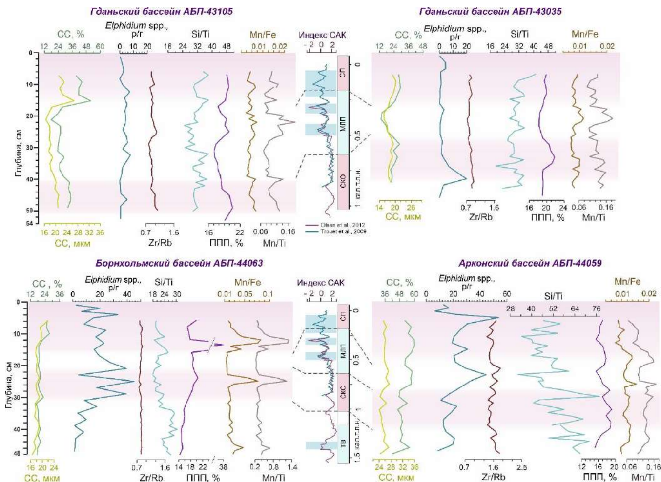
Рисунок 7 — Распределение геохимических, микропалеонтологических и гранулометрических данных в осадочных колонках, полученных в Арконском, Борнхольмском и Гданьском бассейнах. Периоды потепления выделены красным цветом. Климатические события голоцена отмечены на боковой панели: ТВ — Темные века, СКО — средневековый климатический оптимум, СП — современное потепление. CC — сортируемый силт. Вариации индекса САК представлены согласно Olsen et al. (2012), Trouet et al. (2009).
